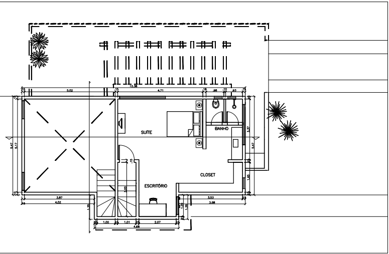
PAVIMENTO SUPERIOR esc 1:100
