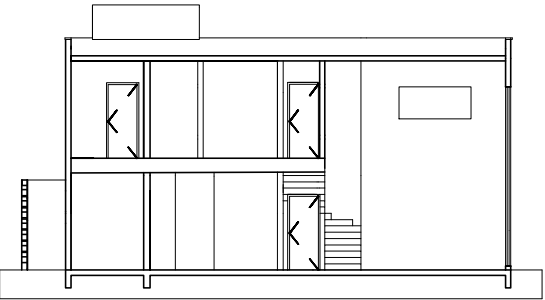
PAVIMENTO SUPERIOR esc 1:100
