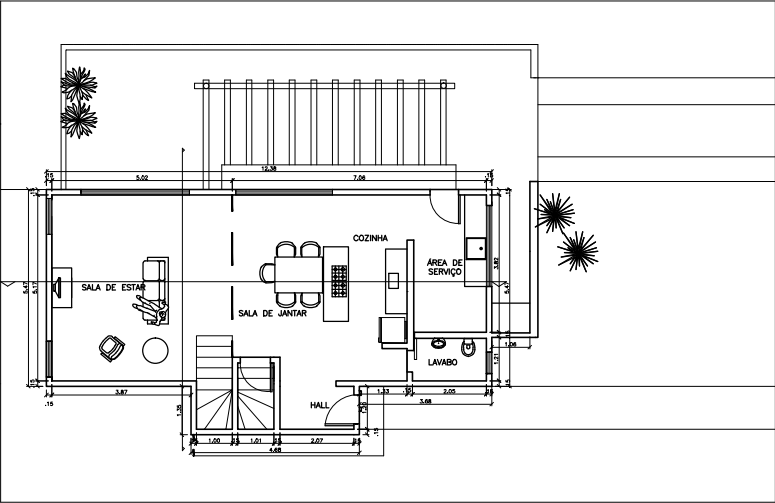
PAVIMENTO TÉRREO esc 1:100
